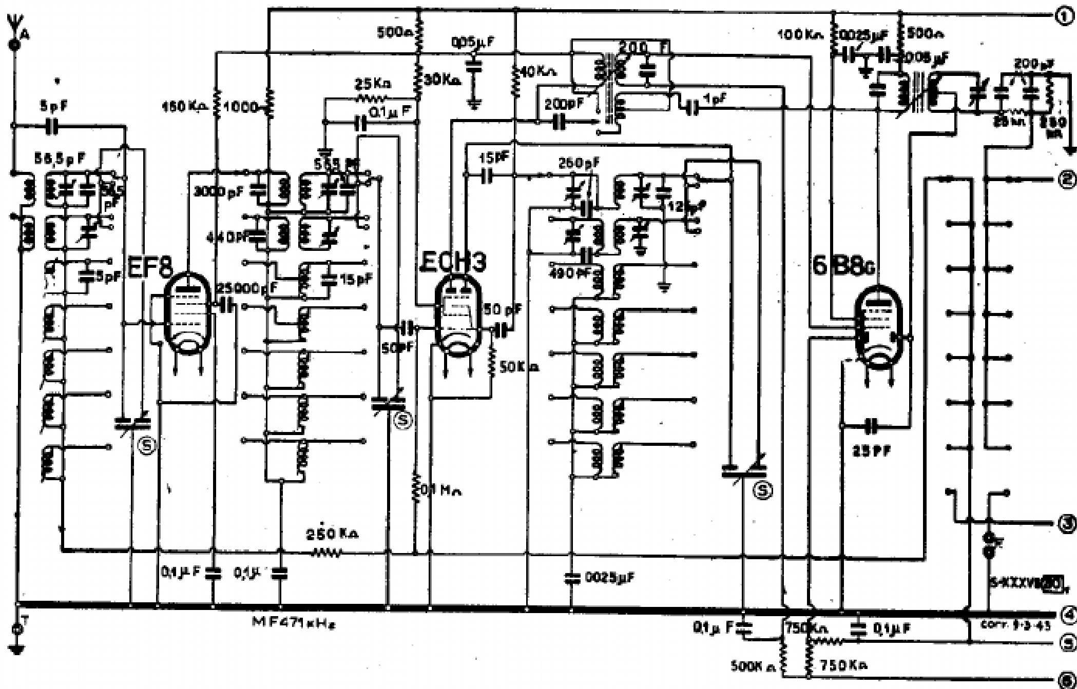
WATT RADIO - MOD. «MONDIALE» - PARTE AF - MF
